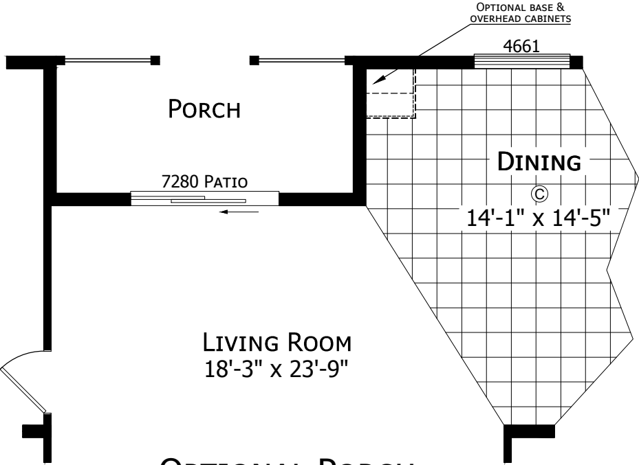
OPTIONAL PORCH
