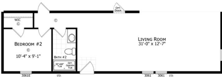
Opt. 2 Bedroom
