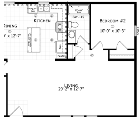
Opt. 2 Bedroom
