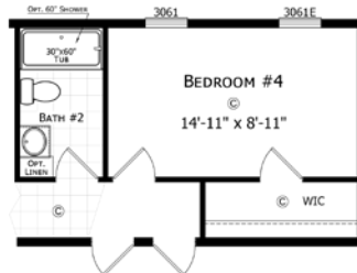
Opt. Bedroom 4
