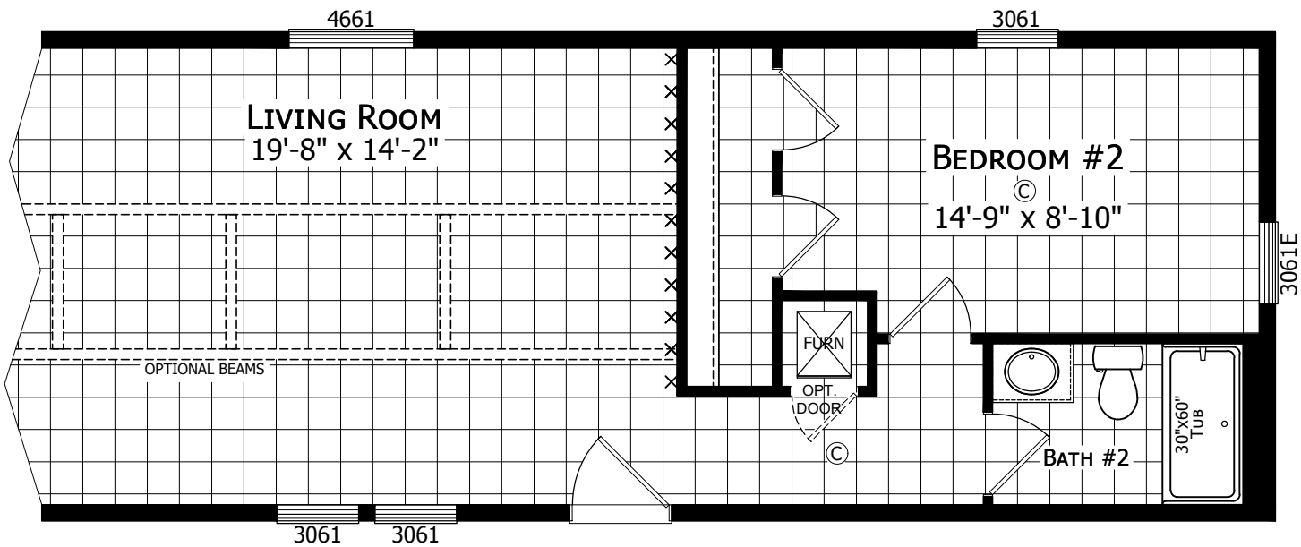
OPTIONAL 2 BEDROOM
